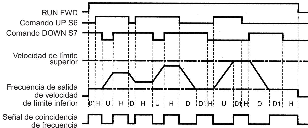
Diagrama de tiempo de introducción de los comandos UP/DOWN
