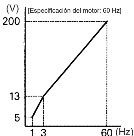
V/f de alto par de arranque
