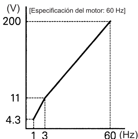
V/f estándar
